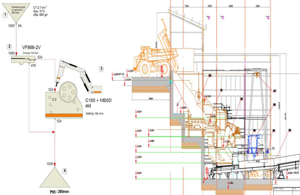
Пресек на примарно дробење
