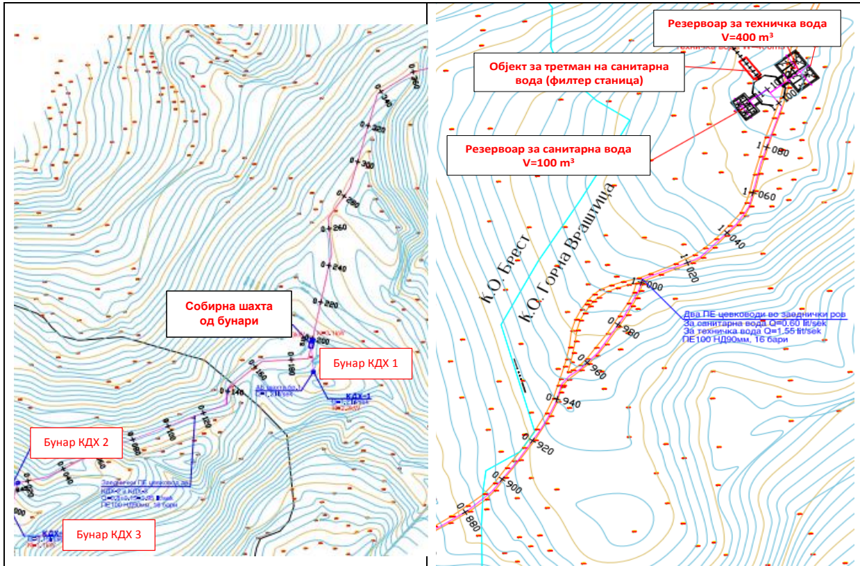
Локација на трите бунари за снабдување со техничка и санитарна вода на рудникот Боров Дол, резервоарите и филтер станицата
