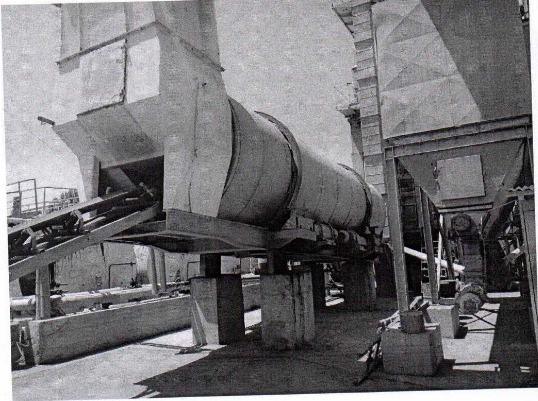
Слика бр.2 – Барабан сушара
