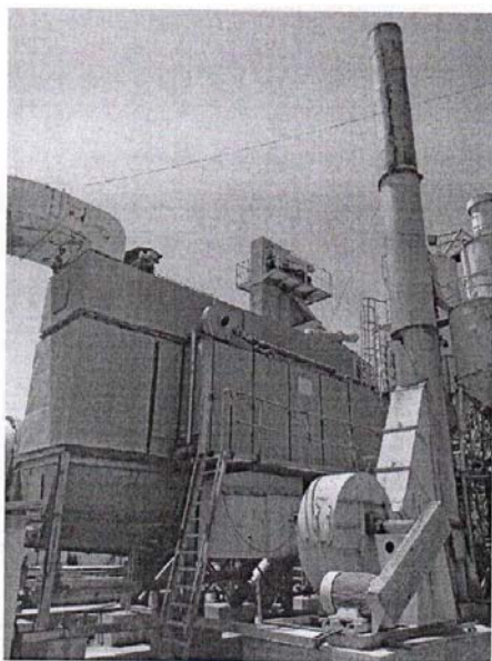
Слика бр.6 – Филтер постројка за суво отпрашување
