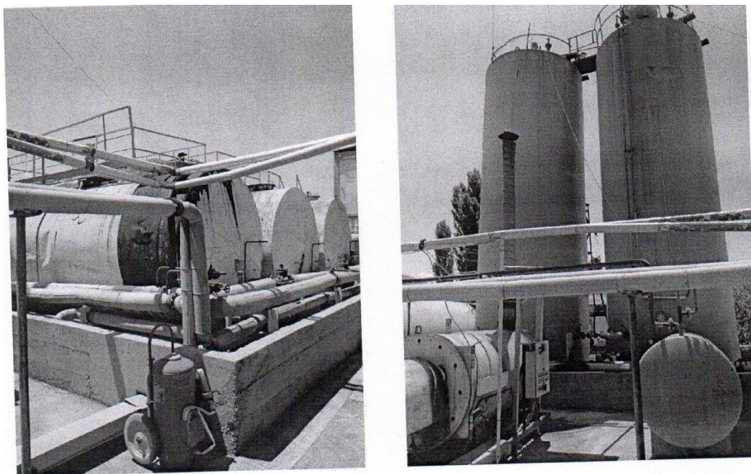
Слика бр.5 – Хоризонтални и вертикални резервоари за битумен
