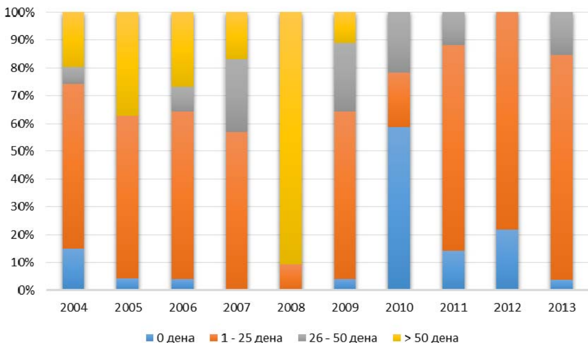
Графикон 2: Процент од урбаната популација изложена на концентрации на ОЗ над долгорочната целна вредност за заштита на човеково здравје, изразена како број на денови во текот на една календарска година
