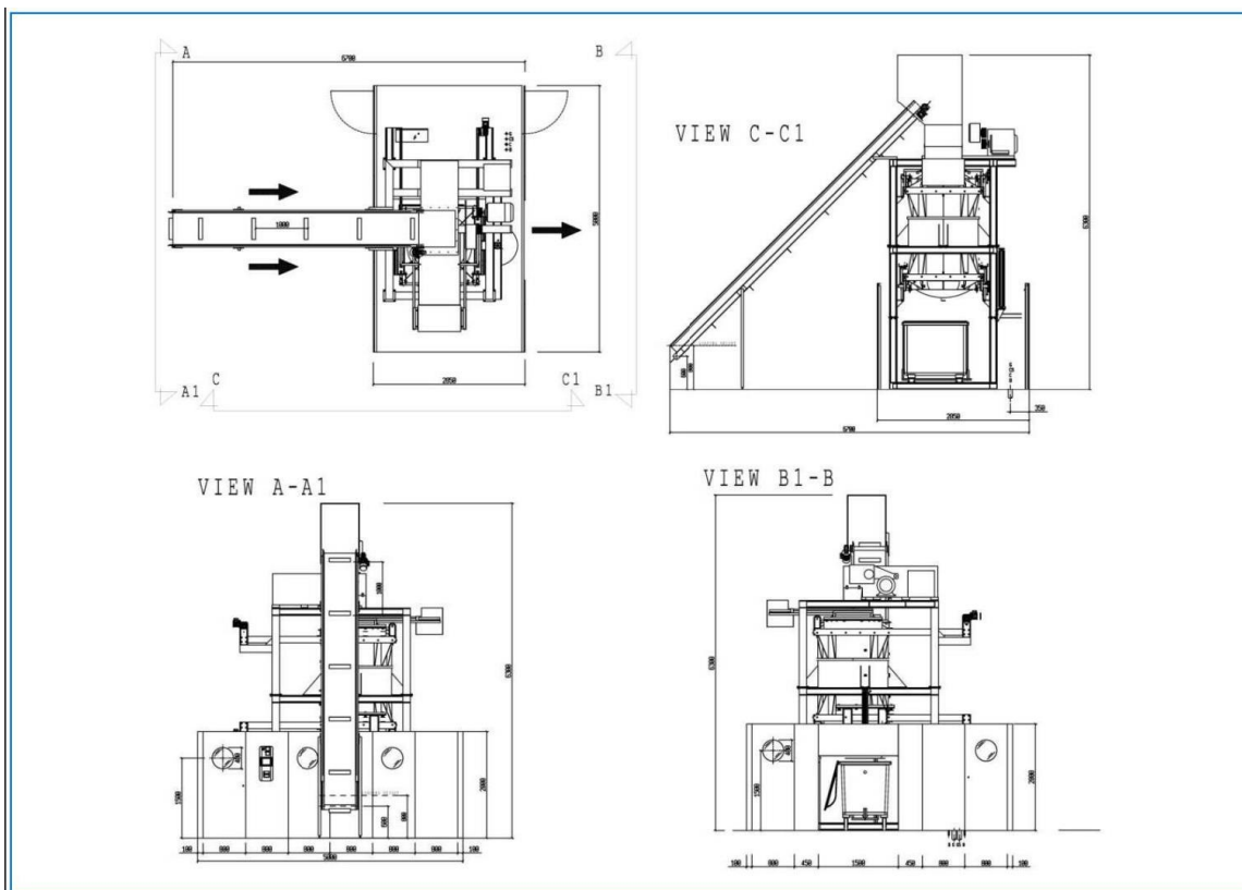
Слика 1. Технички цртеж на постројката за автоклавирање
