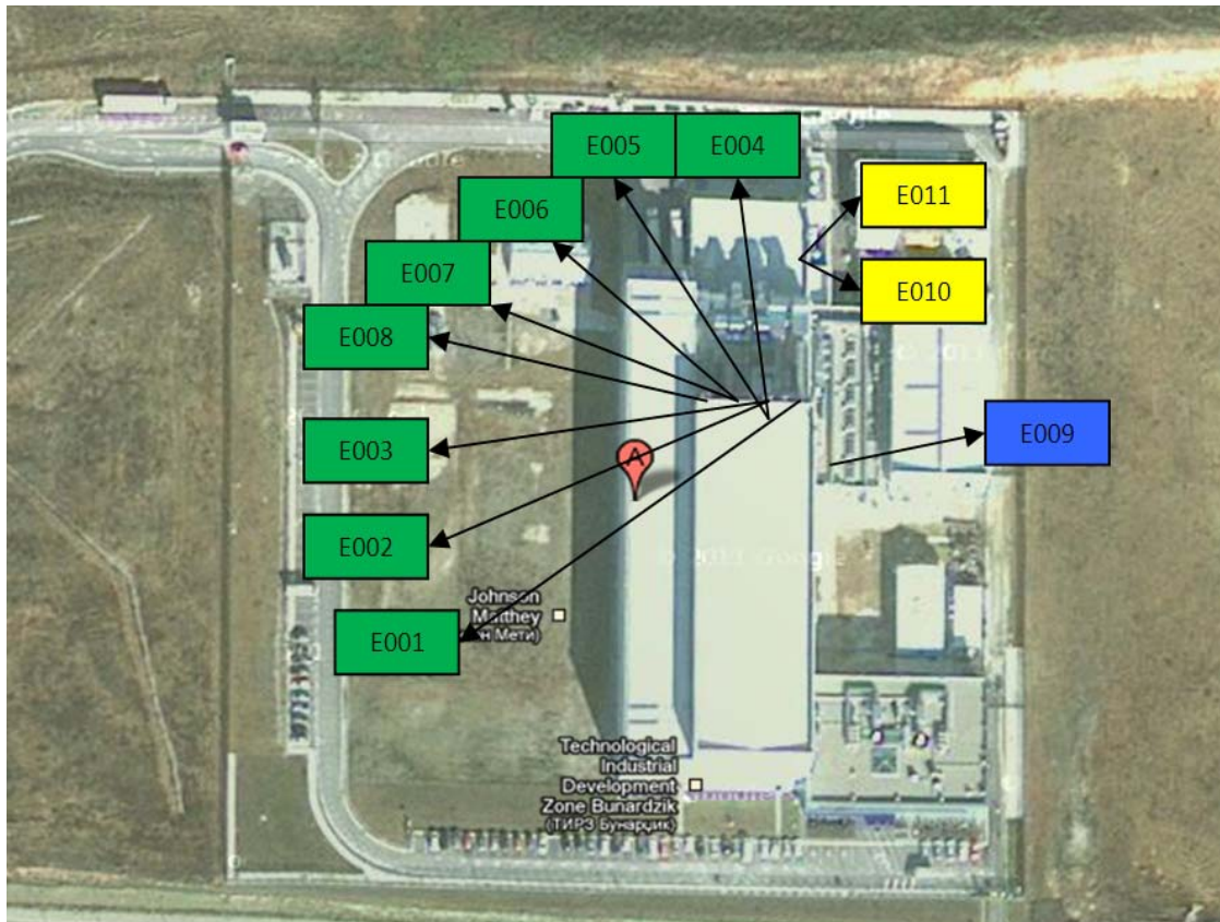
Слика: Шематски приказ на емисионите точки во воздух од страна на инсталацијата за производство на катализатори Џонсон Мети Скопје
